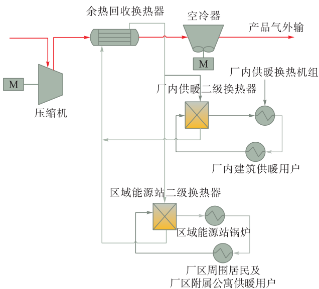
图 2 余热供暖工艺流程图
