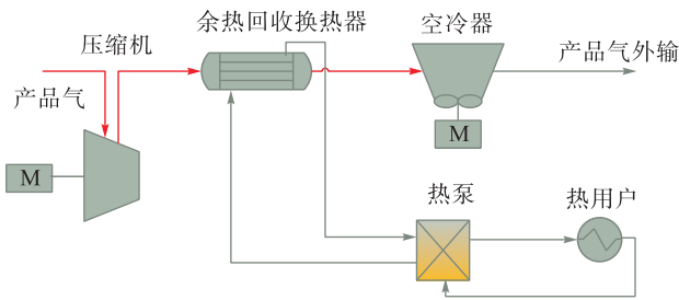
图 1 供热工艺流程图
